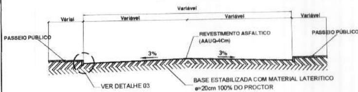
Detalhe 01 - Seção Transversal das Vias
